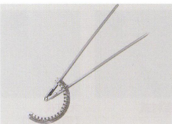
東大式角度計
